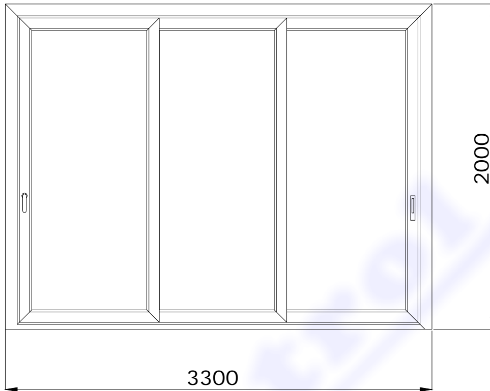
Fig.1a: Prospetto del campione pervenuto e sottoposto a prova (dimensioni nominali dichiarate, espresse in mm)
