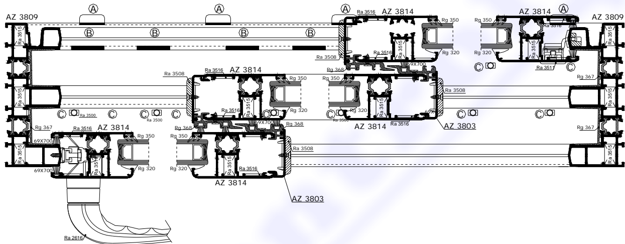
Fig. 2b: sezione orizzontale del campione pervenuto e sottoposto a prova (dimensioni nominali dichiarate, espresse in mm)
