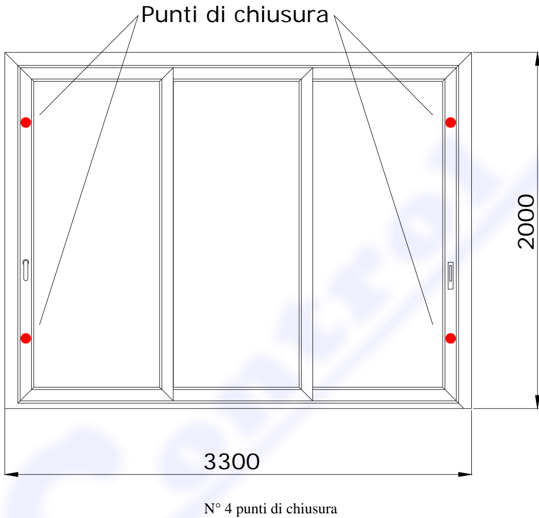
Fig.1b: punti di chiusura del prospetto del campione pervenuto e sottoposto a prova (dimensioni nominali dichiarate, espresse in mm)
