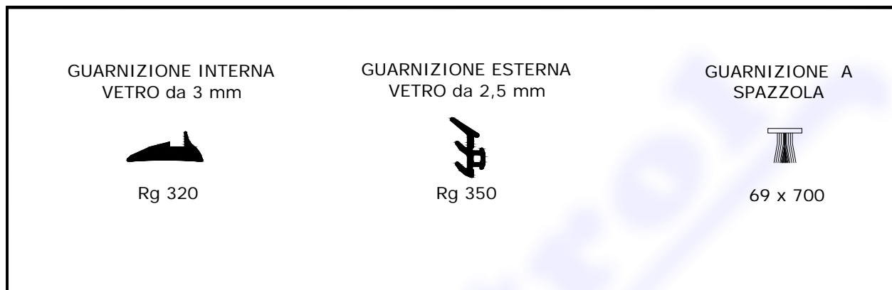
Fig. 4a: Dettagli del sistema di tenuta del campione pervenuto e sottoposto a prova (dimensioni nominali dichiarate, espresse in mm)
